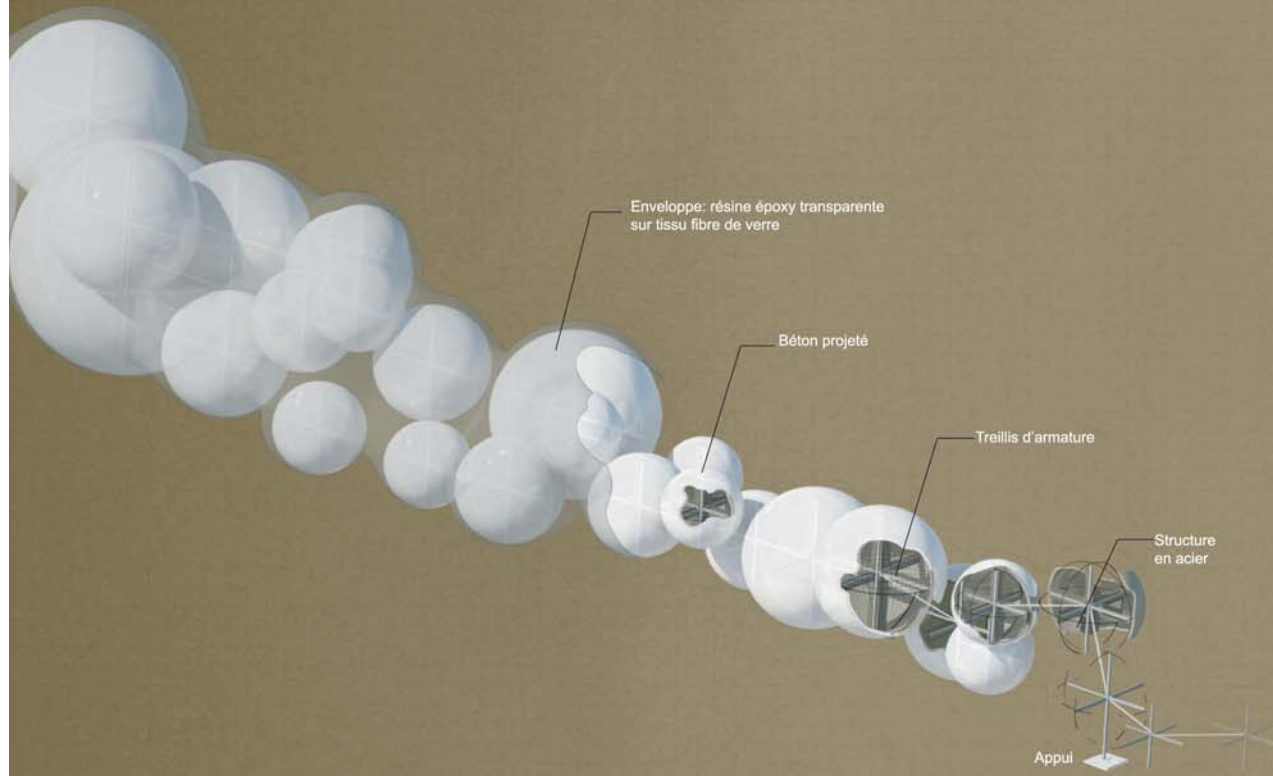
Axonométrie
